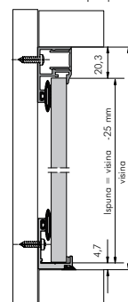
Izračun dimenzija ispune
