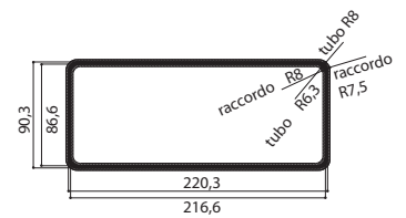
PRAVOKUTNA SPOJNICA 220X90 MM FUN 112.0459.428
